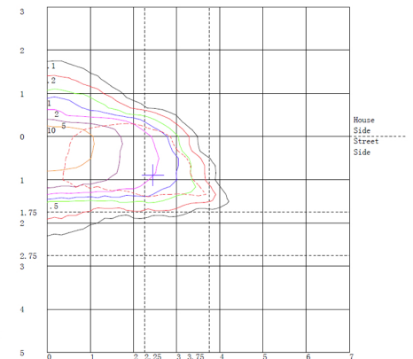
ISO footcandle →
