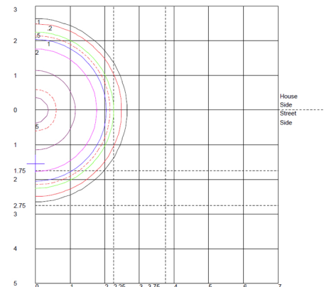
ISO footcandle →
