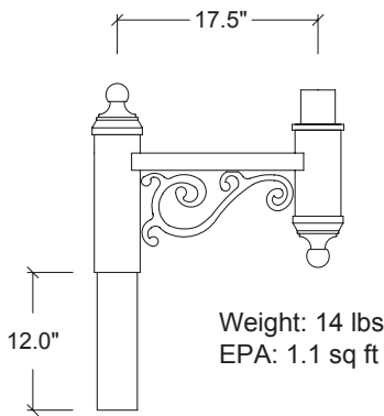
A305 - 1A
