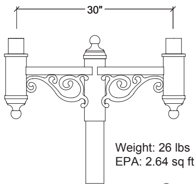
A305 - 3B
